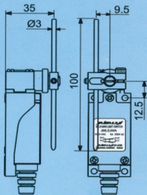
JMLSJWA
