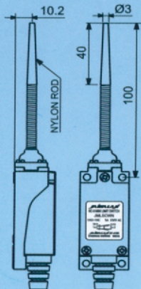
JMLSCWN
