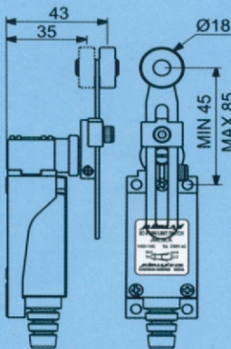
JMLSLA
