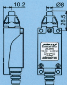
JMLSTPB
