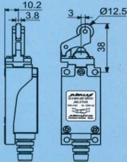
JMLSTNR
