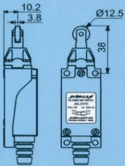
JMLSTPR
