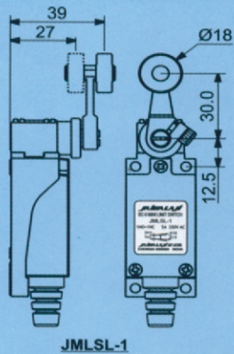
JMLS-1
