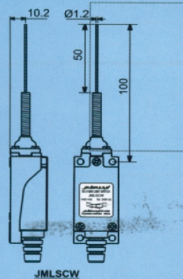
JMLSCW
